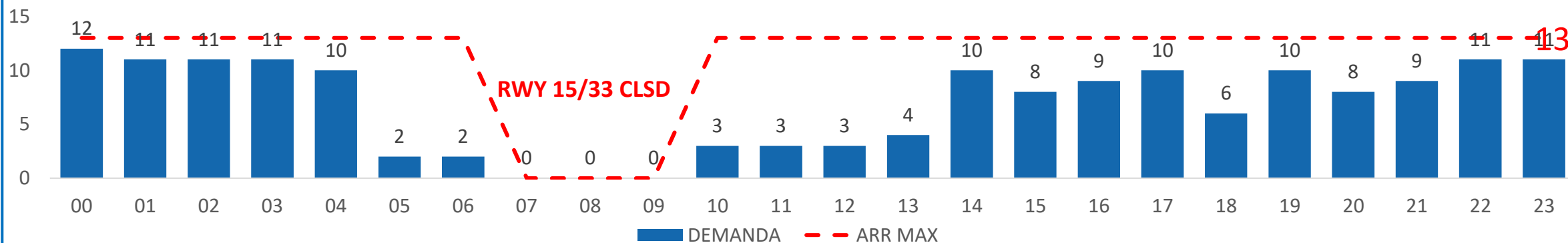
Gráfico de Demanda: 280222 00:00 /280222 23:59 UTC Av. Com. Reg. ARR RWY 15 - SPJC
