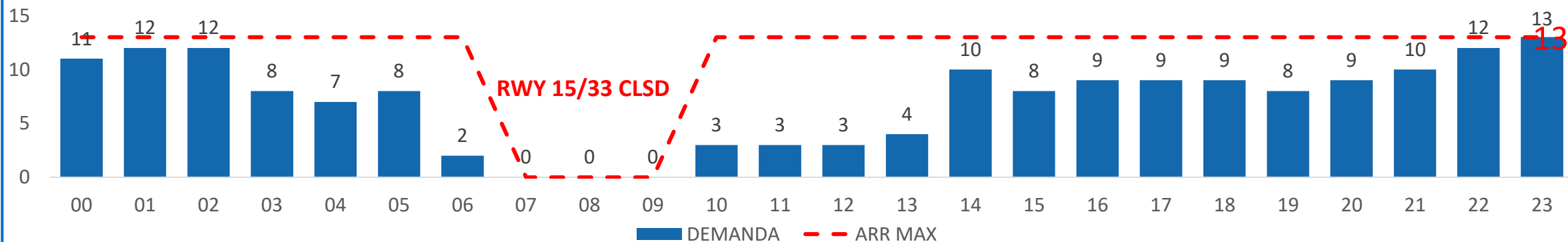
Gráfico de Demanda: 220222 00:00 /220222 23:59 UTC Av. Com. Reg. ARR RWY 15 - SPJC
