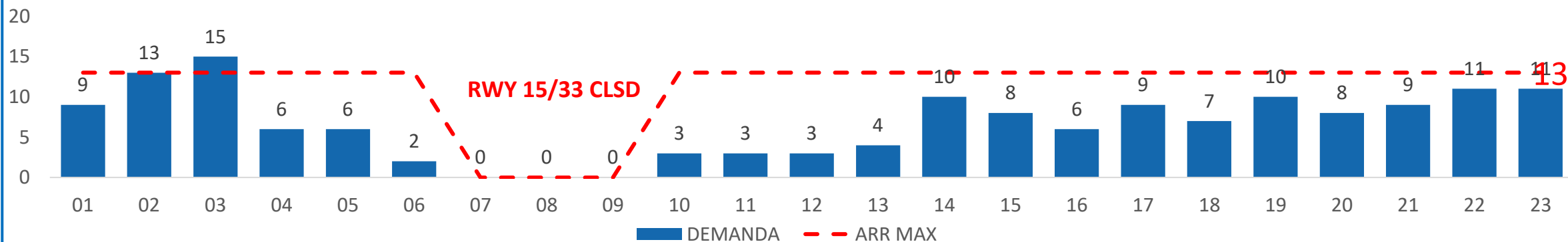
Gráfico de Demanda: 200322 00:00 /200322 23:59 UTC Av. Com. Reg. ARR RWY 15 - SPJC
