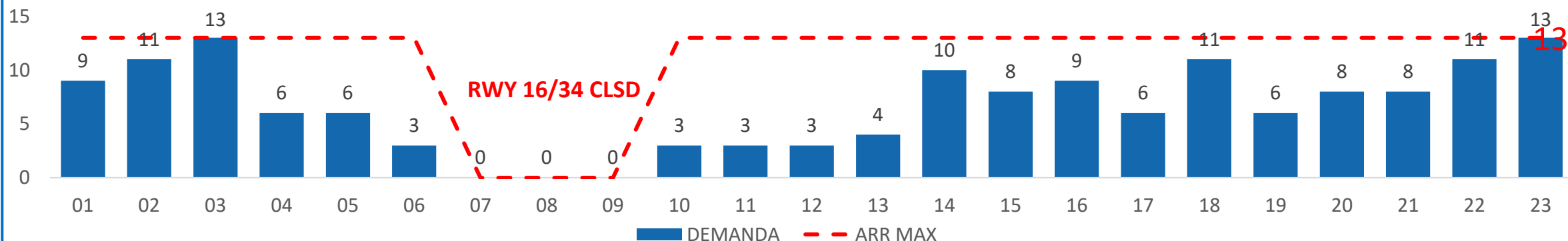
Gráfico de Demanda: 120422 00:00 /120422 23:59 UTC Av. Com. Reg. ARR RWY 16 - SPJC
