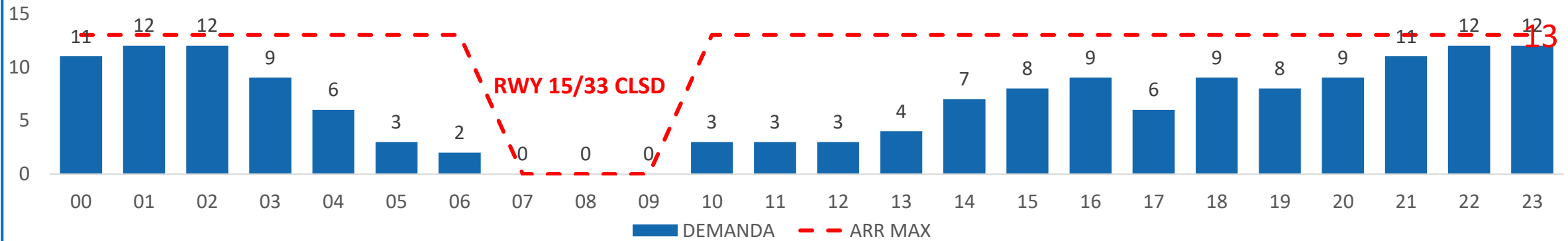
Gráfico de Demanda: 060222 00:00 /060222 23:59 UTC Av. Com. Reg. ARR RWY 15 - SPJC
